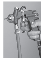
5. Materialschlauch befestigen.
